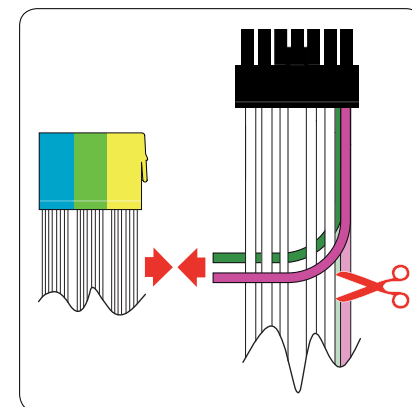
Fig. 06: Connection for the mini ISO connection cable
